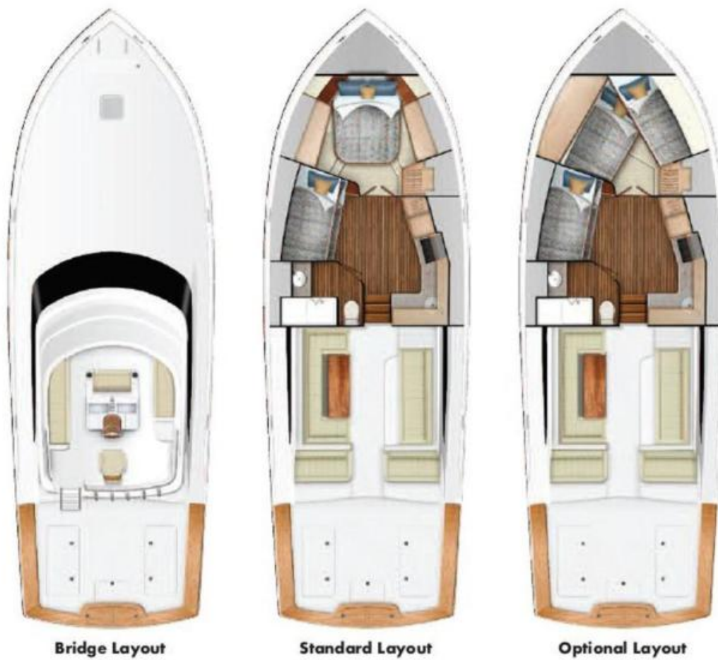
Viking 46- Exterior/Interior Layout Options 2022 Viking 46 Billfish
